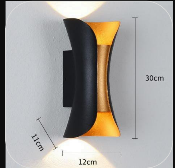
MODEL# NOW328192-BG SIZE: W 11*H30*D12.5cm
